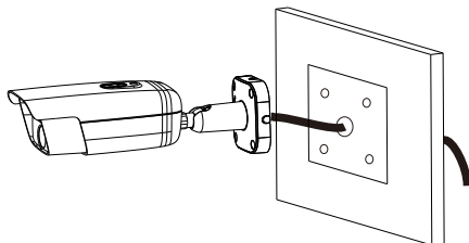
Top wiring
