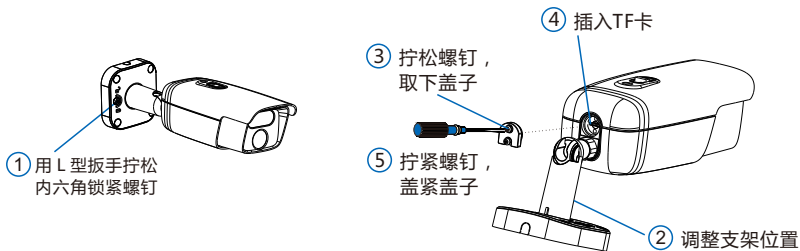
带支架型号TF卡安装
